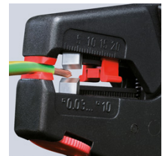
Прецизионное удаление изоляции без повреждения проводника
